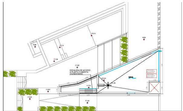
Rooftop – Planta Cubierta
