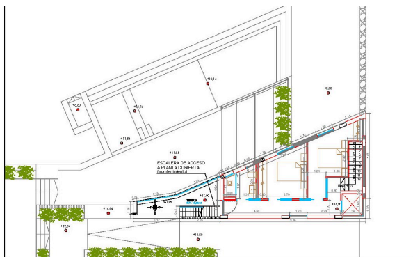
Planta segunda – dormitorios
